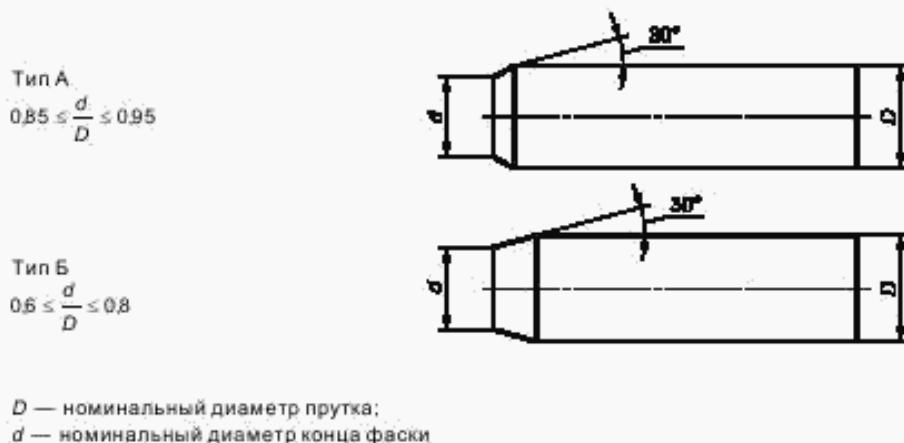
Рисунок 1 — Типы фасок прутков
